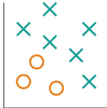
Linealmente separable
